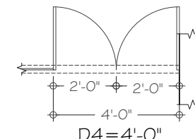
D4 = 4'-0"
