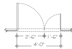
D3 = 4'-0"
